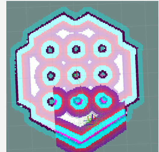
Speed Filter 적용 결과
